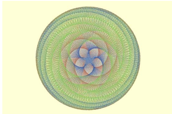
Bewegungsfigur Sonne-Venus-Erde ca. 1358 Jahre
