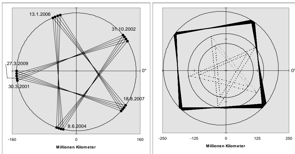
Links: Venus/Erde-Konjunktionen, in der Erdbahn (21 mal), Start 30.3.2001, Zeitraum 31,97 Jahre. Rechts: Mars bei Venus/Erde-Pentagrammen (150 mal), Zeitraum 1199 Jahre; von innen nach außen: Venus-, Erde- und Marsbahn; der Fünfstern ist jeweils nur einmal eingezeichnet. Heliozentrische Darstellungen, Maßstab in Millionen km.
