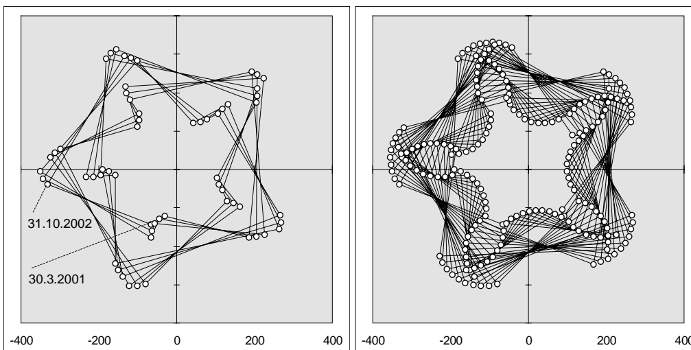
Links: 60 mal, Zeitraum ca. 95,9 Jahre; rechts: 200 mal, Zeitraum ca. 319,7 Jahre
